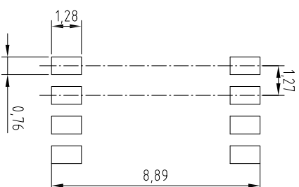
焊盘尺寸:
