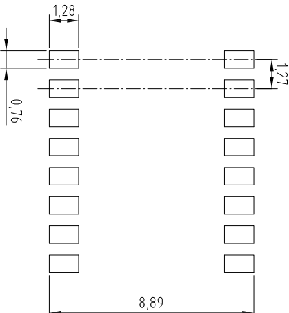
焊盘尺寸:
