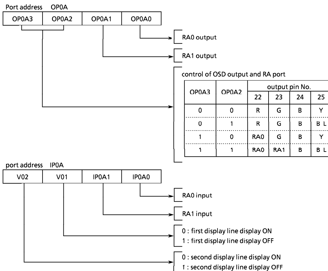
Figure 3-8. Port RA
